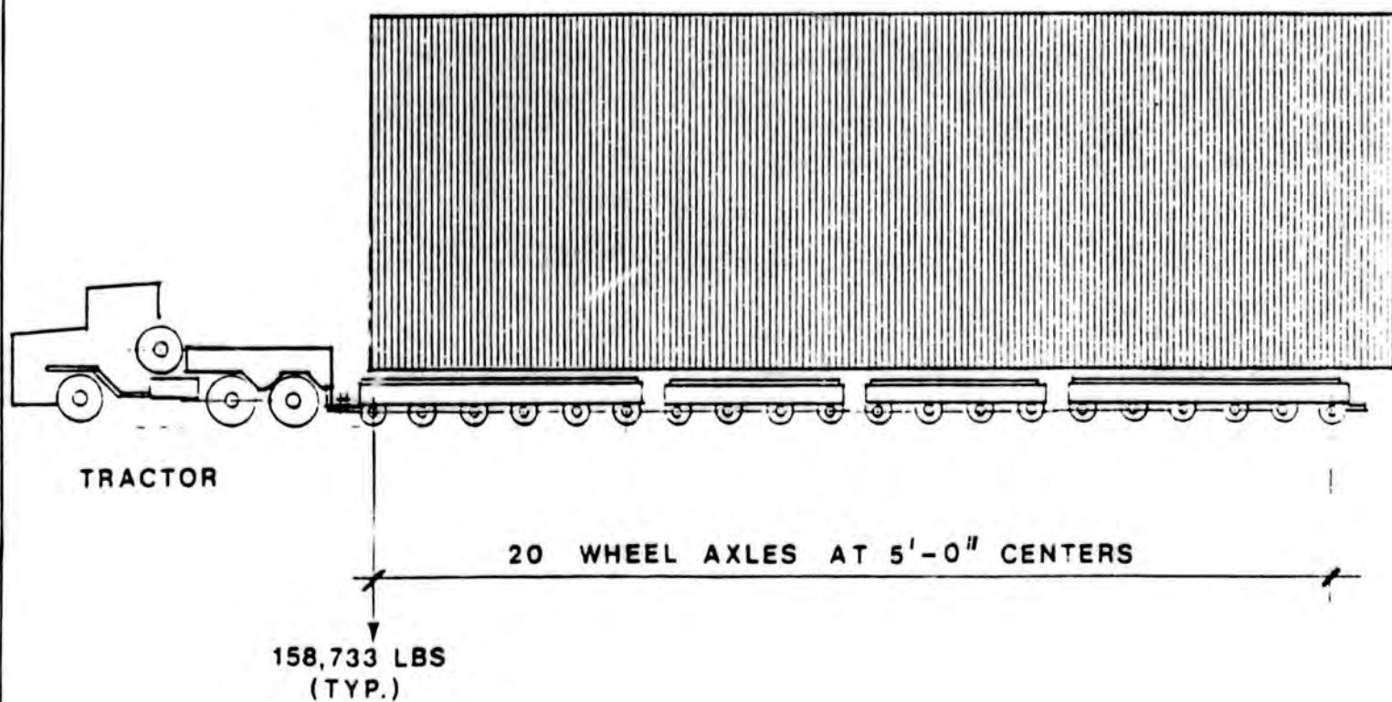
MODULE TRANSPORTER
